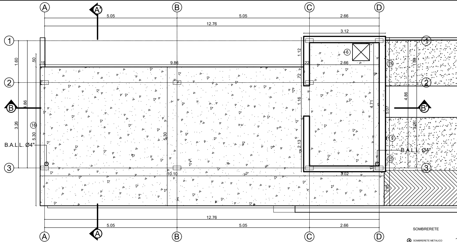
PLANTA DE CUBIERTAS ESC:1/25
